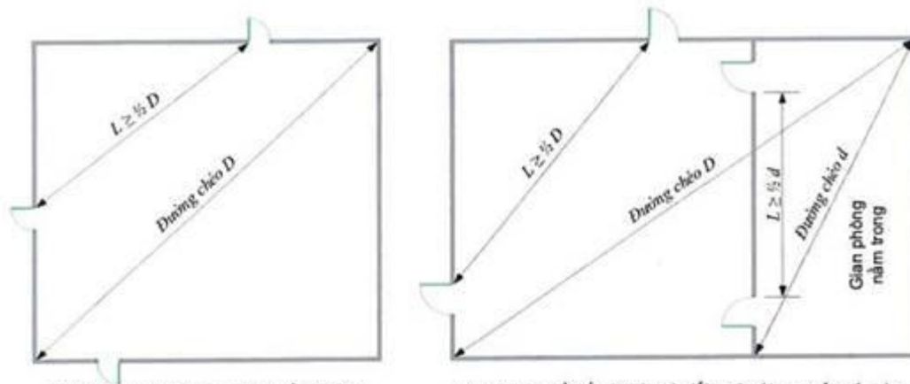
a) Minh họa về bố trí phân tán lối ra thoát nạn của một gian phòng, một phần nhà hoặc một tầng nhà
