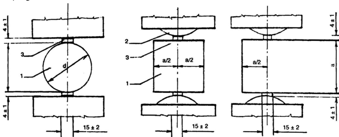
Hình 1. Sơ đồ thử bừa a. Mẫu trụ ; b. Mẫu lập phương ; c. Mẫu dầm.
