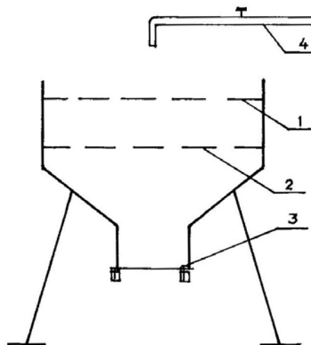
Hình 1 : Sơ đồ dụng cụ thử thành phần hỗn hợp bê tông 1. Sàng 5mm; 2. Sàng 1,2mm; 3. Sàng 0,15mm; 4. Ống dẫn nước
