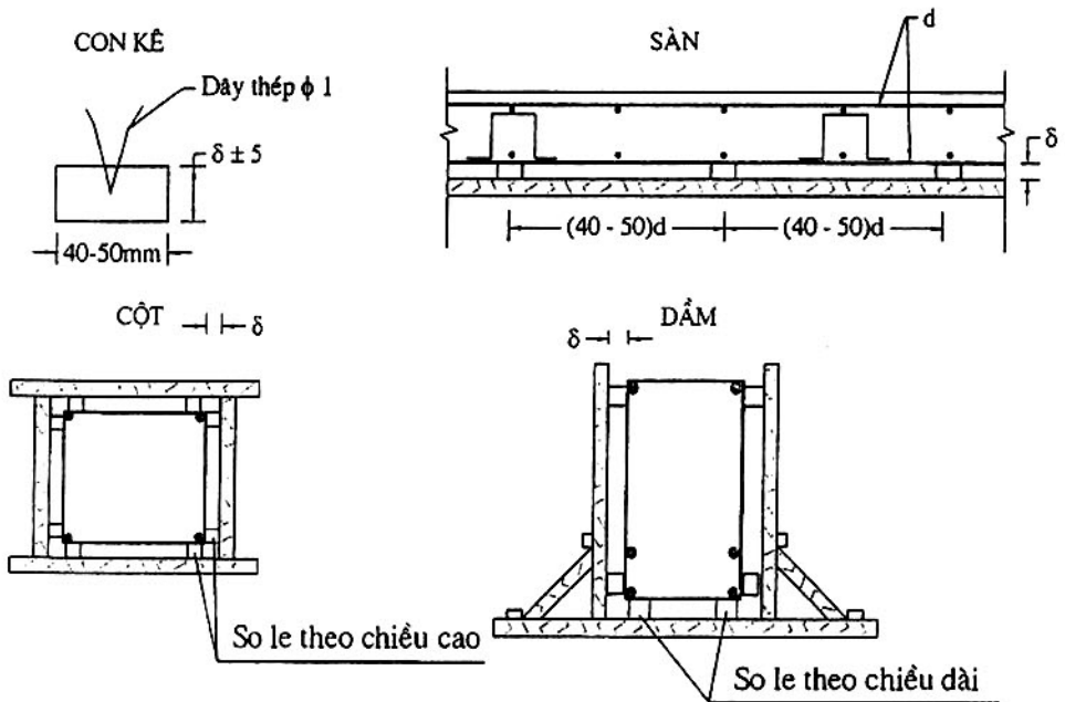
Hình 1 - Cách đặt các con kê
