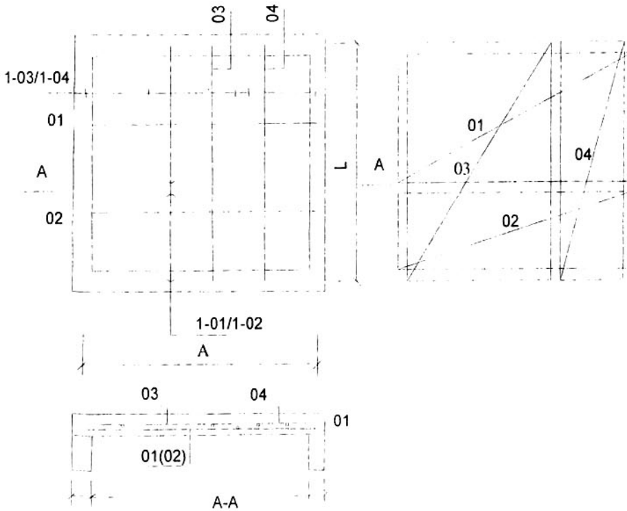
Hình E.6 - Lưới thép trong sàn chịu lực 2 phương, gói đơn giản
