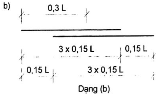
Hình E.4: Lưới thép bố trí thành hai lớp để chịu mô men âm ở vùng gối của sàn
