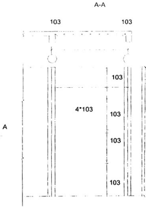
Hình E.2 - Lưới thép đặt đơn giản trong sàn chịu lực một phương, kê tự do
