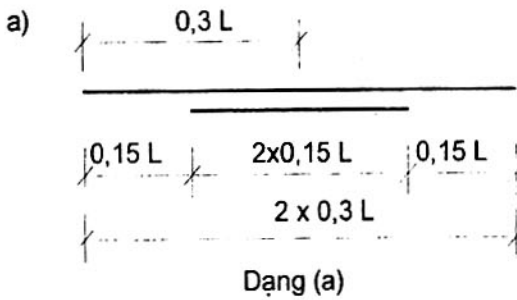
Hình E.4: Lưới thép bố trí thành hai lớp để chịu mô men âm ở vùng gối của sàn
