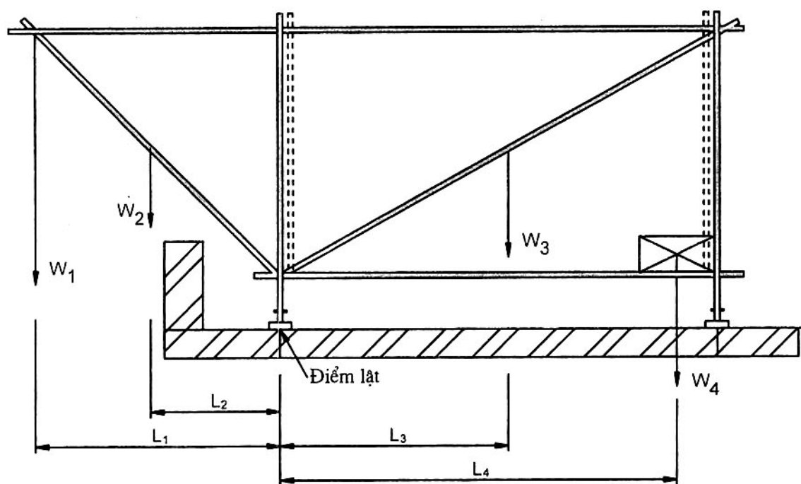
Hình 1 – Sơ đồ tính toán ổn định của giáo treo
