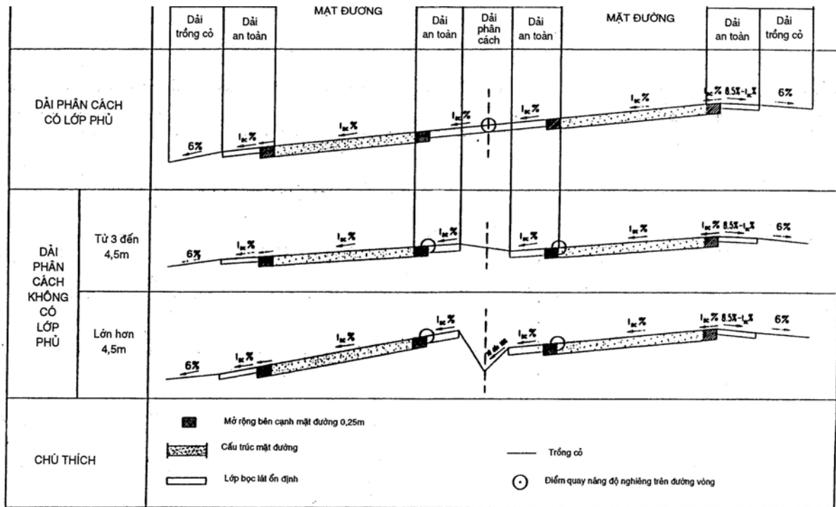
Hình 3.: Độ dốc ngang của mặt đường
