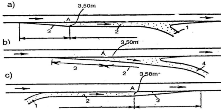
Hình 5 : Các giải pháp bố trí chỗ ra, vào đường cao tốc
