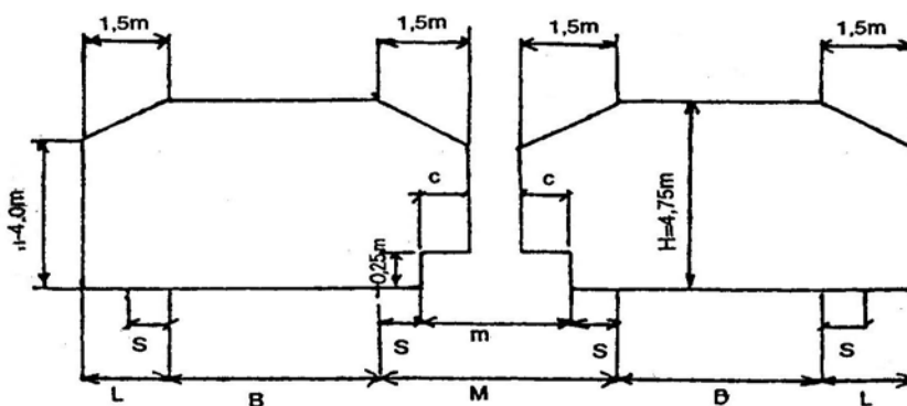
Hình 1 : Giới hạn tĩnh không trên đường cao tốc
