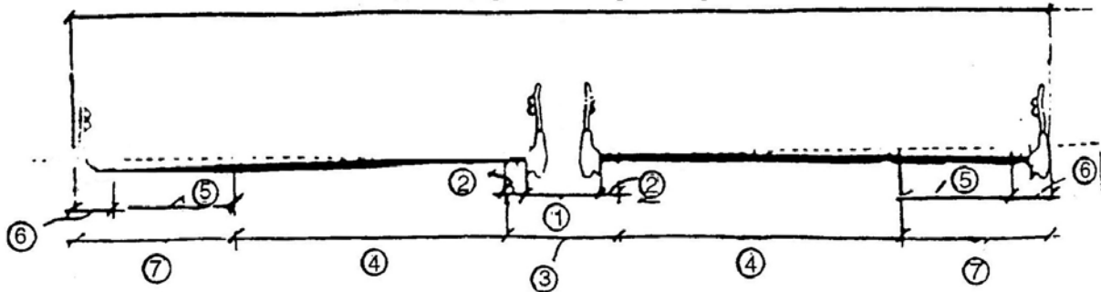
Hình 4: Mặt cắt ngang cầu trên đường cao tốc
