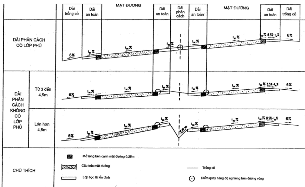
Hình 3.: Độ dốc ngang của mặt đường
